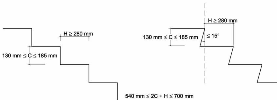
FIGURA 4.2. CONFIGURACIÓN DE LOS PELDAÑOS
