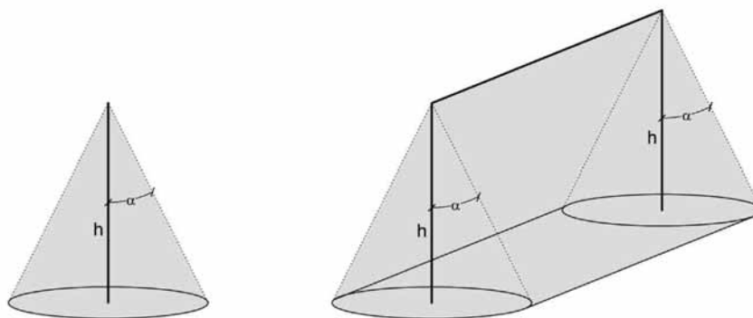
FIGURA B.1. VOLUMEN PROTEGIDO POR CAPTADORES
