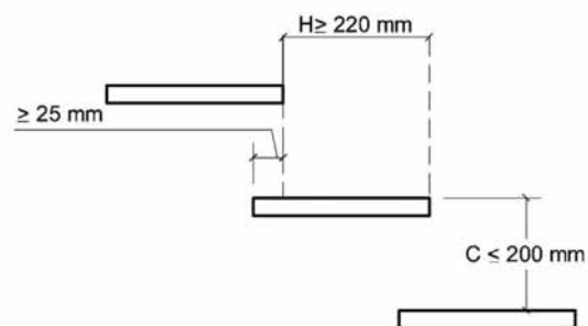
FIGURA 4.1. ESCALONES SIN TABICA
