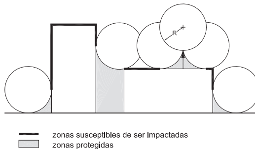
Figura B.3 Esfera rodante en estructuras
